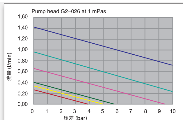
G2-026 性能曲线
