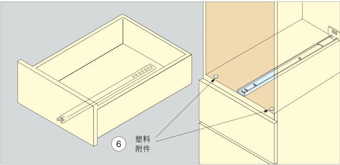
安装示意图
