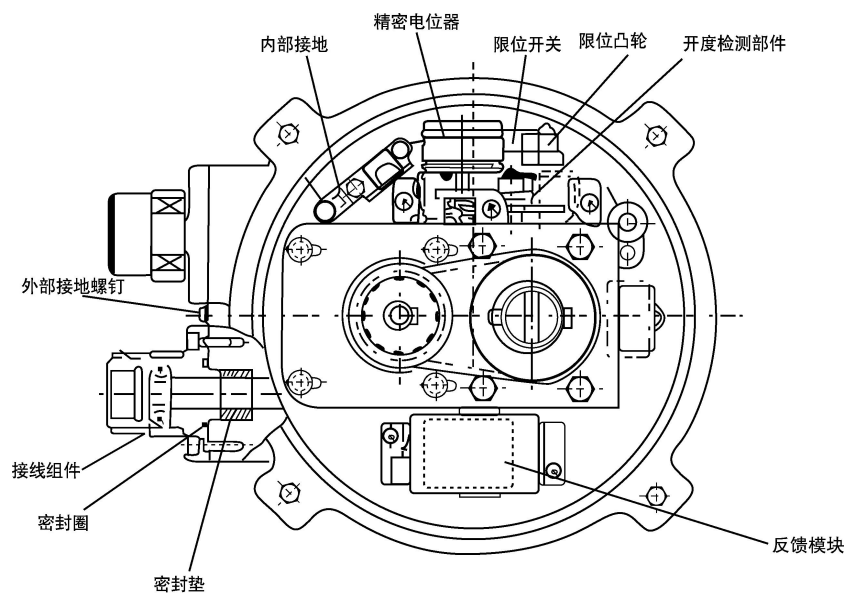
图4 381LXA、381LXB型执行器
