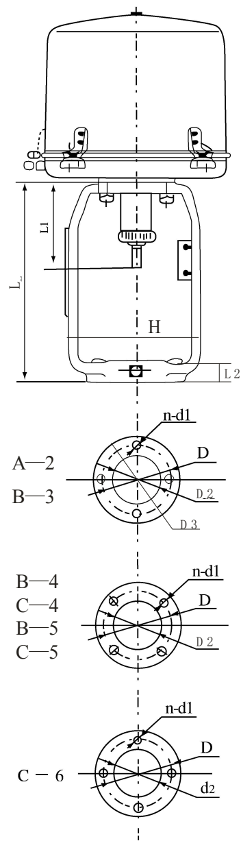
图12 支架与阀门连接螺栓孔尺寸
