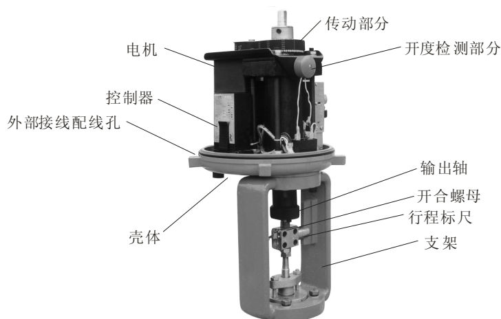
图1 执行器外观
