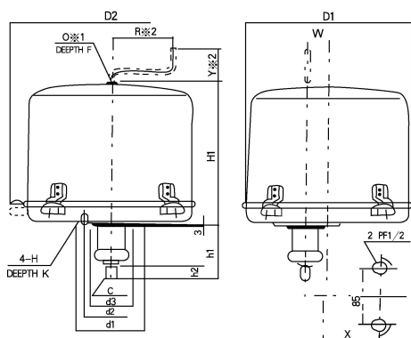
图10 381LSA、381LSB型
