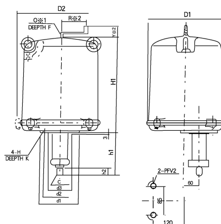
图11 381LSC型
