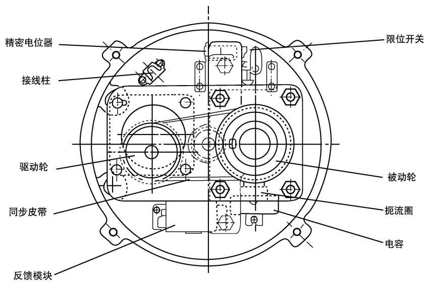
图3 381LSC型执行器
