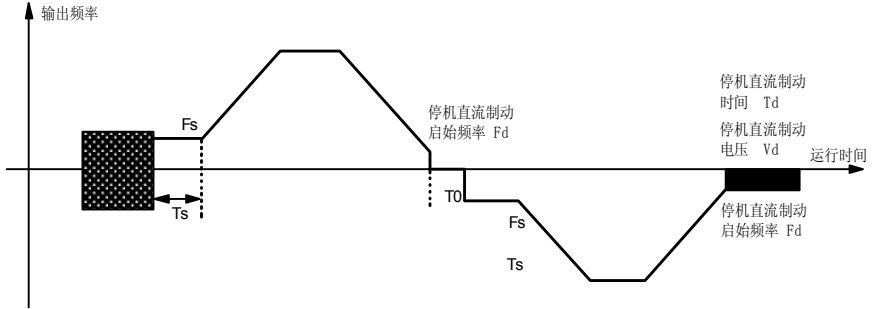
6.2.1 启动方式1（正转、反转运行及停机）示意图
