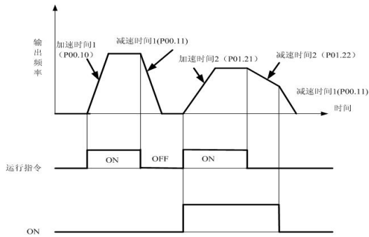
图 6.1.10 两种加减速时间的切换
