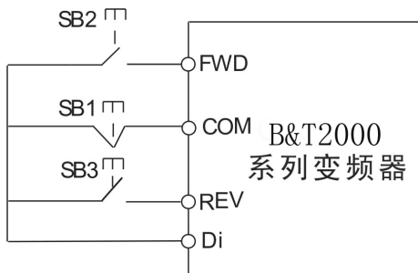
图 6.2.12 三线控制模式 2
