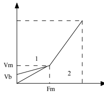
图 6.1.6 折线 V/F 曲线
