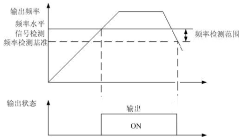
图6.2.15 输出频率 \geq 频率检测基准
