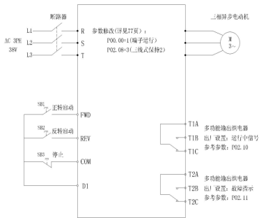
图七：三线式保持控制方式
