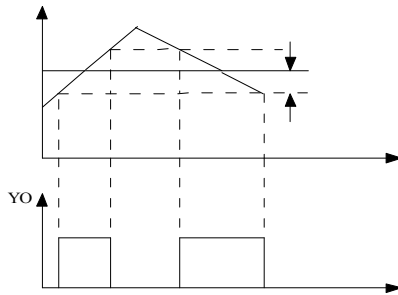
图6.2.13 频率到达信号及频率到达检出宽度示意图
