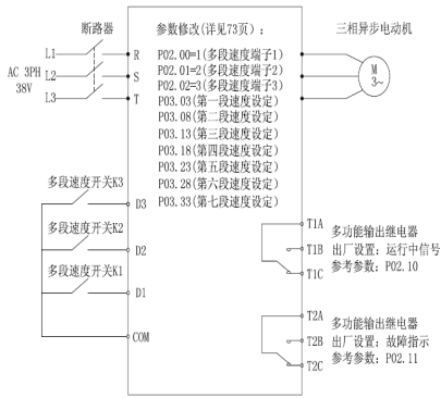
图五：变频器多段速控制图
