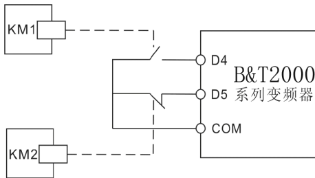
图 6.2.8 外部设备故障常开/常闭输入示意图
