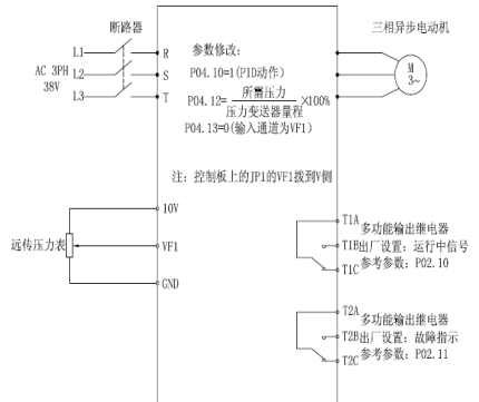
图四：恒压供水 PID 控制图（远传压力表）
