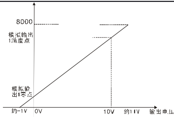
图6.2.17 模拟输出零点1及满度点1
