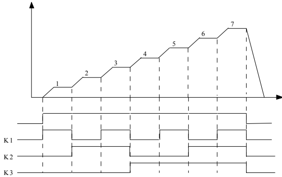
图6.2.7 多段速度运行示意图
