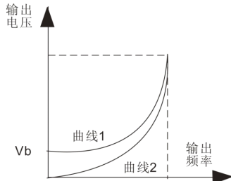
图 6.1.5 递减转矩模式 2
