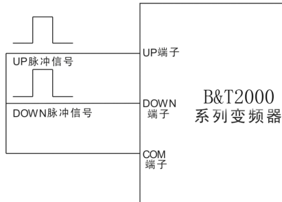
图 6.1.2 频率给定 10、11 方式时，接线示意图
