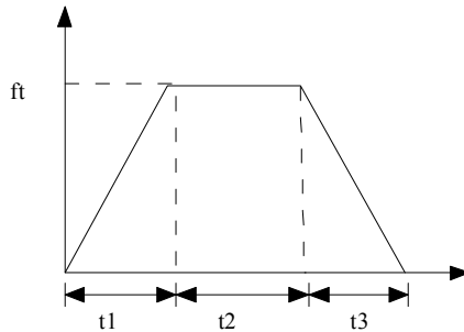
图6.2.4 点动运行参数说明
