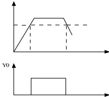
图6.2.14 频率水平检出信号示意图
