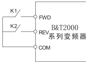
图6.2.9 两线控制模式 1
