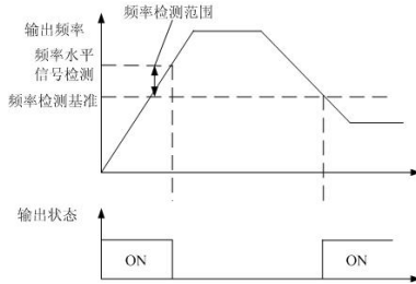
图6.2.16 输出频率≤频率检测基准
