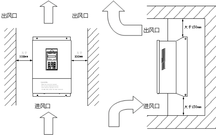
B&T2000 系列变频器的安装空间
