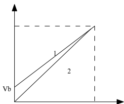
图 6.1.3 恒转矩 V/F 曲线
