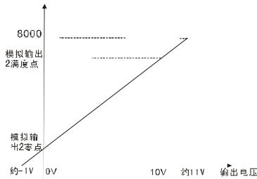
图6.2.18 模拟输出零点2及满度点2
