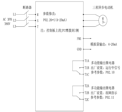
图六：变频器 4-20mA 输出图
