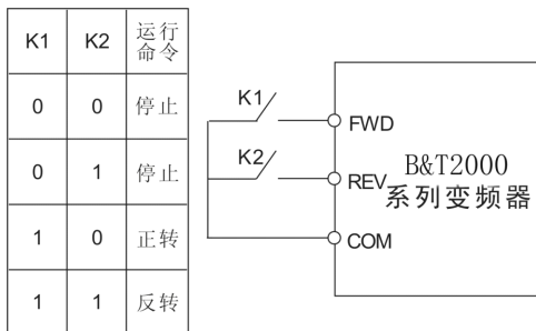
图 6.2.10 两线控制模式 2
