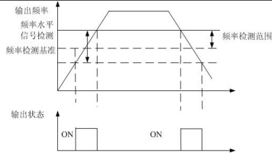
图6.2.16 输出频率=频率检测基准
