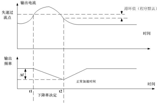
图6.4.3 恒速中失速过流保护
