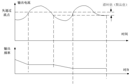
图6.4.1 过压失速功能示意图
