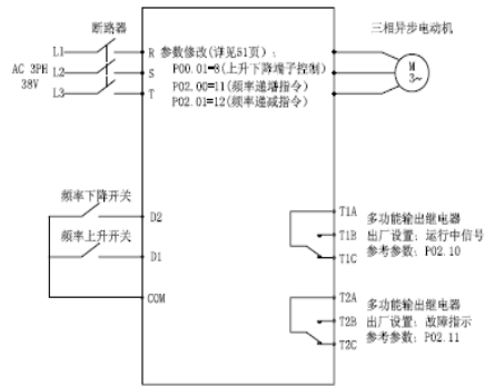
图二：上升/下降端子控制频率
