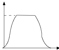
图 6.1.8 S 曲线加减速
