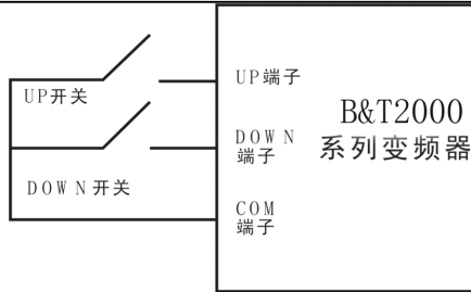
图6.1.1 频率给定8、9方式时，接线示意图
