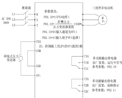
图三：恒压供水 PID 控制图（压力变送器）
