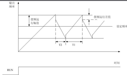
图 6.3.2 变频运行图
