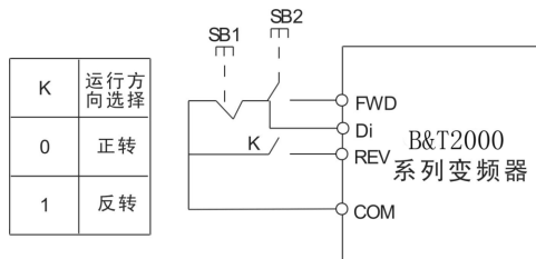
图 6.2.11 三线控制模式 1
