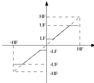
图6.1.11 极限频率参数定义示意图
