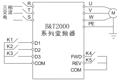
图6.2.6 多段速度运行接线图
