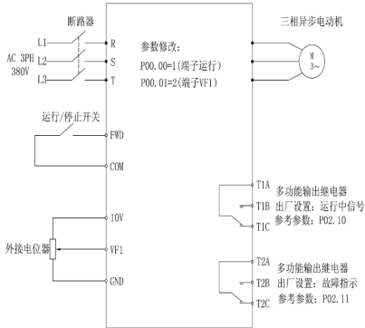
图一：外部启停、外部电位器调速图
