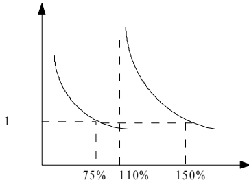
图6.1.12 过载保护反时限特性曲线
