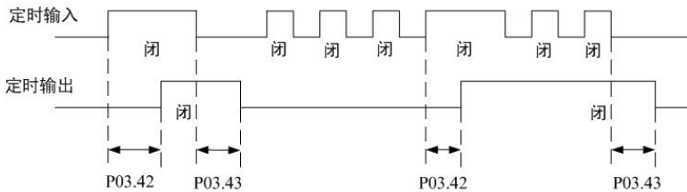
图 6.3.3 定时器功能图
