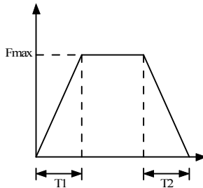
图6.1.9 加、减速时间的定义
