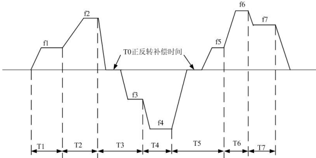
图6.3.1 可编程多段速运行示意图
