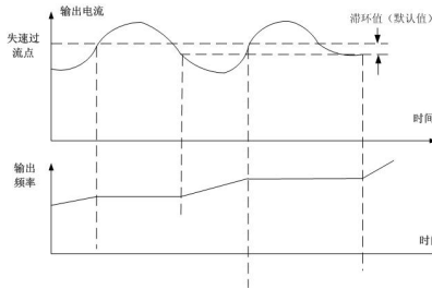
图6.4.2 加速中失速过流保护
