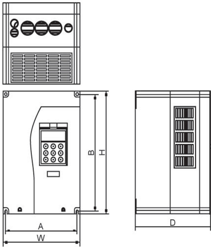
B&T3100S 外形安装尺寸
