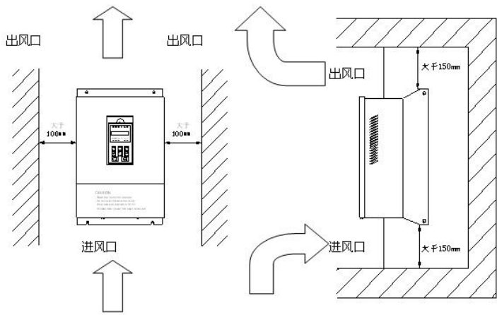
B&T 系列变频器的安装空间
