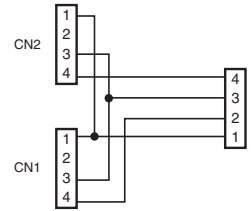
配线图
