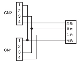
配线图
