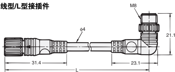
L型/直线型接插件
