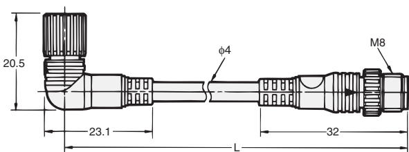
L型/直线型接插件
