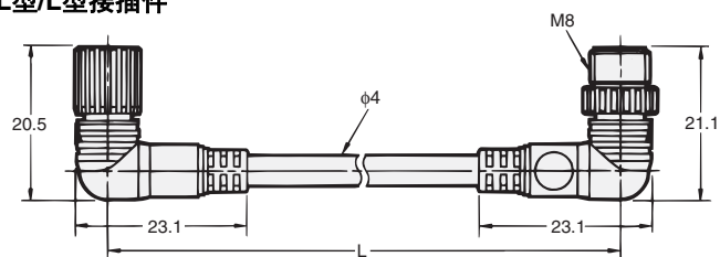
L型/L型接插件
