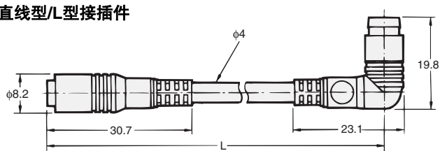
直线型/L型接插件
