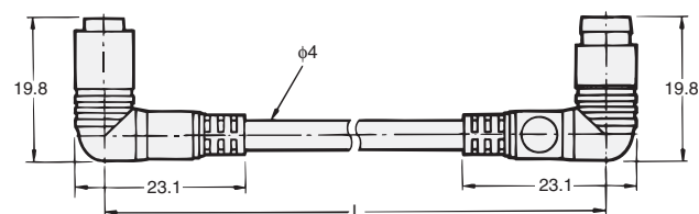
L型/L型接插件
