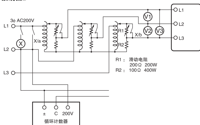
接线图2
