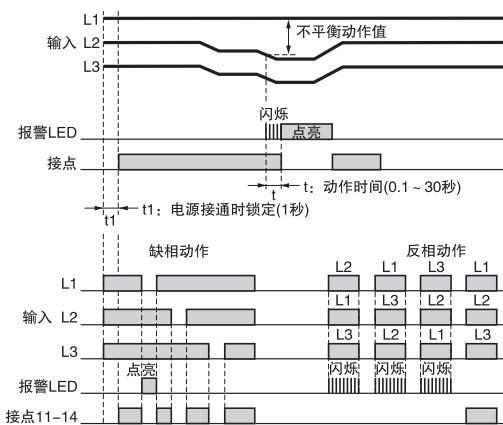
电压不平衡与反相缺相动作的说明图
