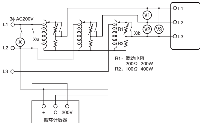
接线图2
