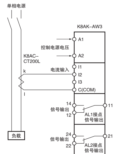
〈K8AK-AW3时〉
