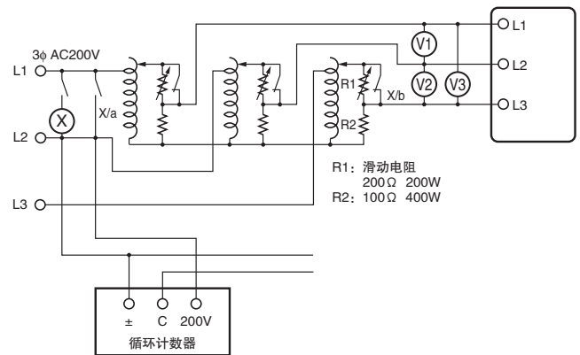
接线图2
