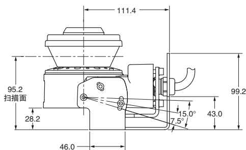
侧视图
