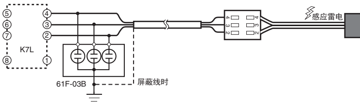
61F-03B 电极连接端子侧
