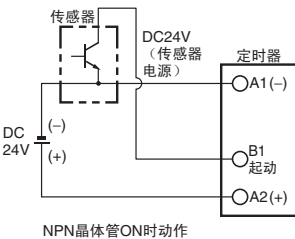
NPN晶体管ON时动作
