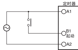
接点ON时动作
