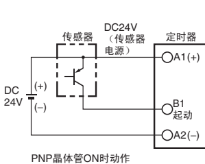
PNP晶体管ON时动作
