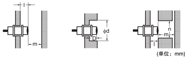
两倍距离型 <屏蔽型>
