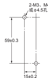
安装孔加工尺寸 (顶视图)
