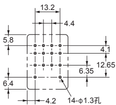
印刷电路板加工尺寸
