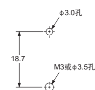
安装孔加工尺寸 (顶视图)
