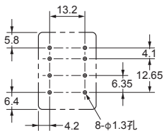
印刷电路板加工尺寸
