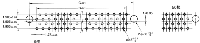
印刷基板加工尺寸 (BOTTOM VIEW) 40、60、80、100极
