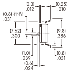
端视图
