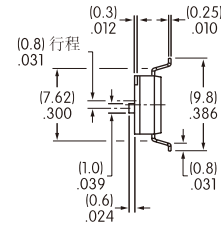
端视图
