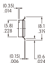
端视图
