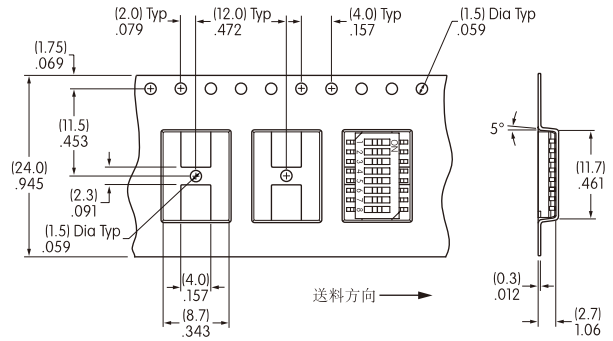
用于JS0408FP4-R的磁带尺寸
