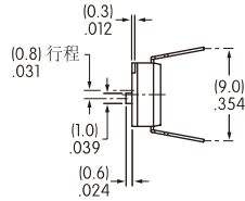
端视图
