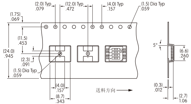
用于JS0404FP4-R的磁带尺寸
