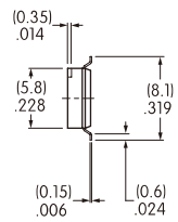
端视图
