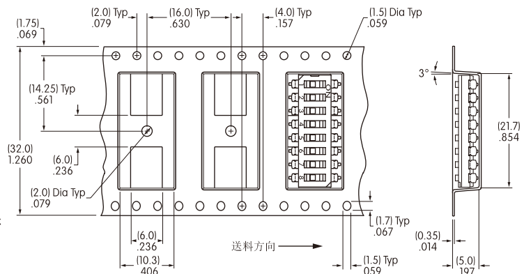
用于JS0208AP4-R的磁带尺寸
