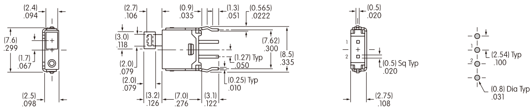
单极
