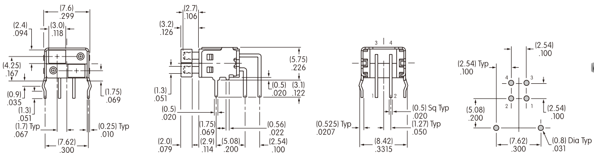
单极带2个开关
