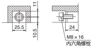
端子部详图
