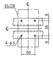
安装开孔尺寸 (角铁安装时)
