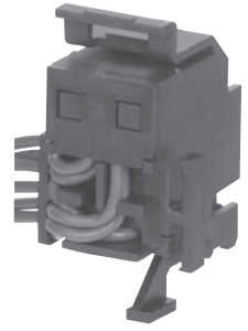
辅助开关+报警开关 (WK)
