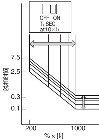
电流设定范围, 额定电流 I_1 的200%~1000%。
