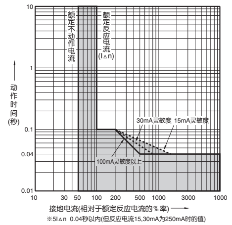
●漏电脱扣特性
