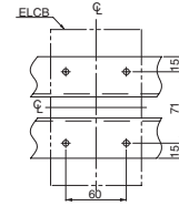
安装开孔尺寸(角铁安装时)
