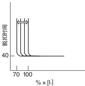
预报警电流设定范围, 额定电流 I_1 的70%~100%。预脱扣报警动作时间, 40s恒定。
