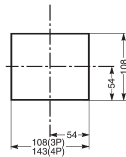
开孔B
