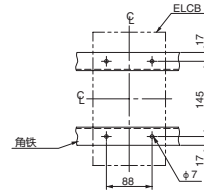
安装开孔尺寸(角铁安装时)
