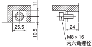
端子部详图
