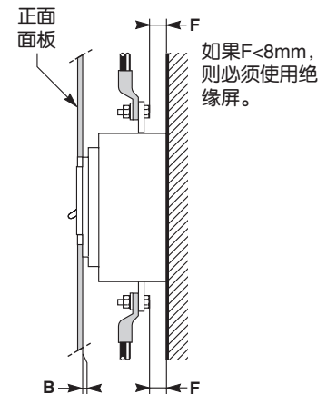
MCCB与正面面板之间的最小距离
