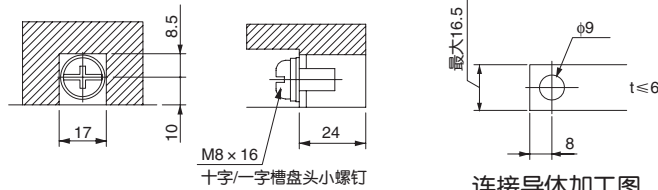
端子部详图
