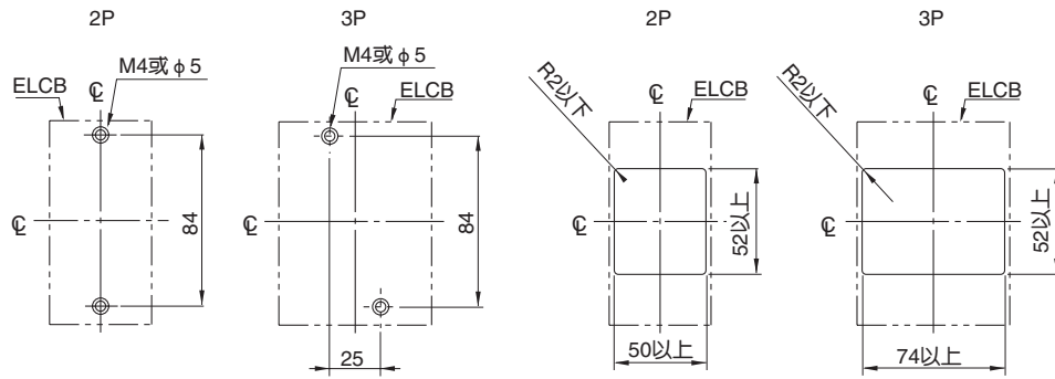
安装孔尺寸
