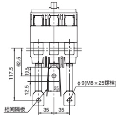
【从电源侧看】
