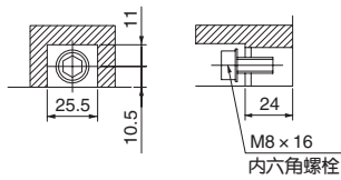
端子部详图
