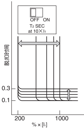
电流设定范围, 额定电流 I_1 的200%~1000%。
