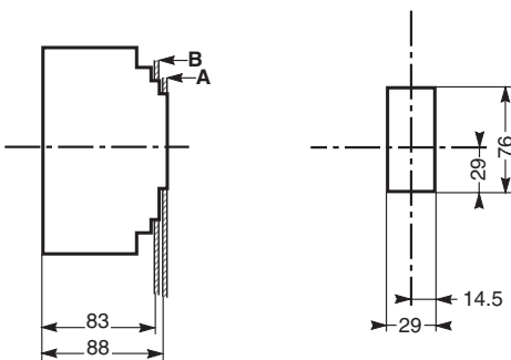
开孔A
