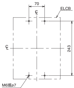
安装开孔尺寸
