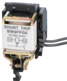
分励脱扣装置
