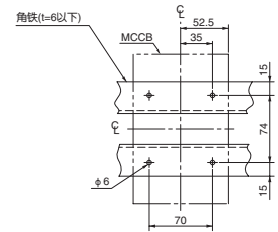
安装开孔尺寸(角铁安装时)
