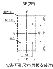
安装开孔尺寸(面板安装时)
