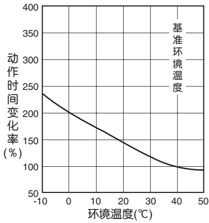
●温度补偿曲线
