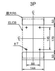
安装开孔尺寸(面板安装时)
