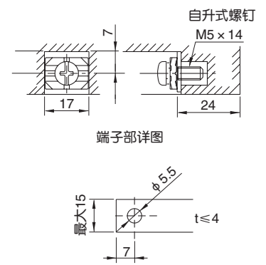
连接导体加工图
