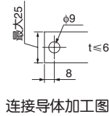
连接导体加工图
