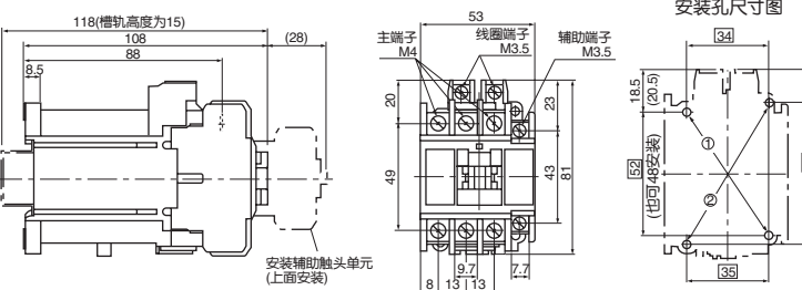
安装孔尺寸图
