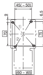
安装孔尺寸图
