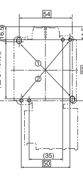
安装孔尺寸图
