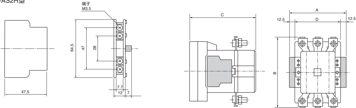
· 尺寸表
