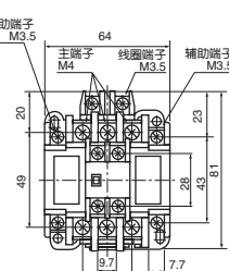
安装尺寸图
