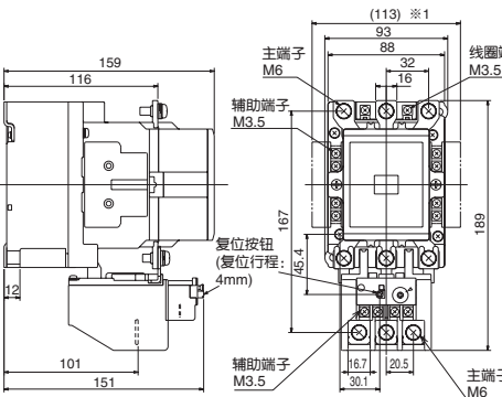
※侧面安装2个辅助触头单元时
