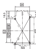
安装尺寸图
