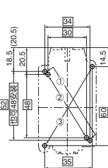
安装尺寸图
