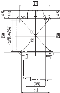
安装孔尺寸图
