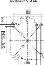
安装尺寸图
