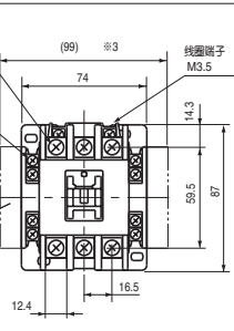
安装尺寸图
