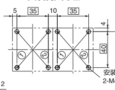
安装孔尺寸图
