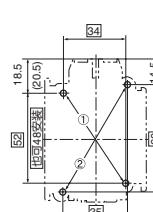
安装尺寸图
