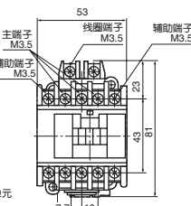
安装尺寸图
