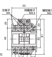
安装尺寸图
