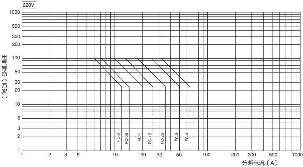
■ AC-3分断电流和电气寿命的曲线图
