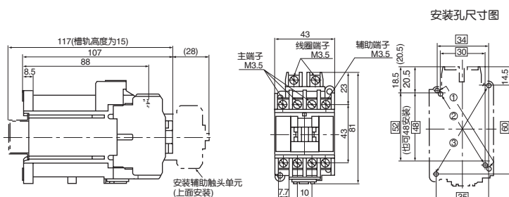
安装孔尺寸图
