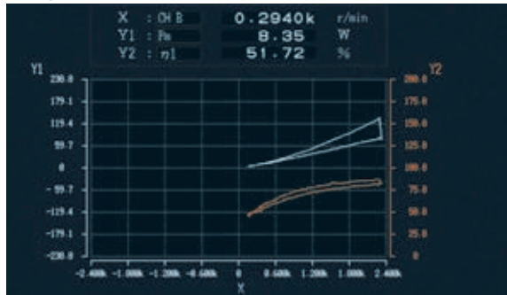
用于评估变频器的特性和制作扭矩图。选择任意项目，可显示 X-Y 曲线图。
