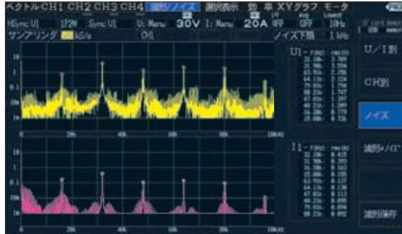
电压和电流的 FFT 结果可用图标及数值显示，最高到 100kHz。最适用于变频器的频率分析。
