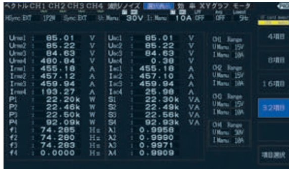
可在项目数 4/8/16/32 的各个画面分别选择显示项目，汇总 1 个画面进行确认
