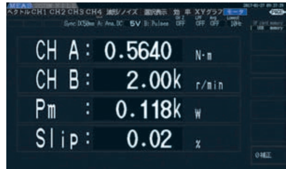
马达分析画面(扭矩、转速、马达功率、转差率)
