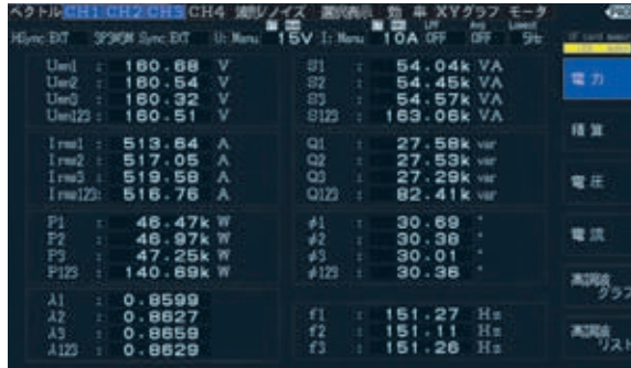
基本测量画面按照接线显示电压 / 电流 / 功率 / 功率因数 / 频率等各种参数的一览表。
