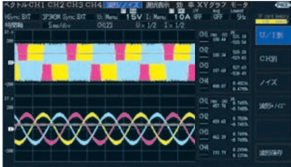
可将 4ch 的电压 / 电流波形，以最快 500kS/s, 外加最长 5 秒显示。可保存波形数据。
