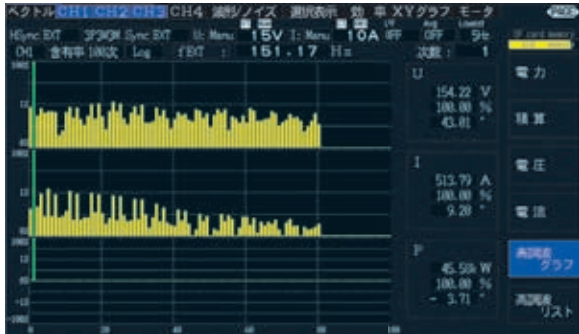
电压 / 电流 / 功率可显示最高 100 次的谐波柱状图。所选择的次数的数值数据也能同时确认。
