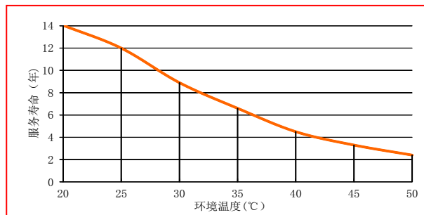
不同温度下的浮充服务寿命曲线
