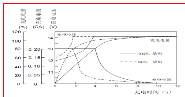
不同放电深度下的充电曲线
