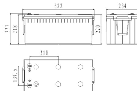
外形尺寸
