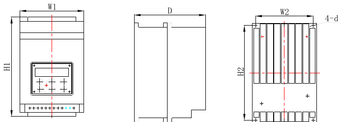
图 3.4 55KW 及以下产品外形图
