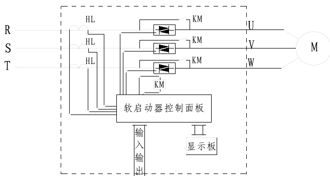
图 7.1 电气原理图 (55KW 以下)
