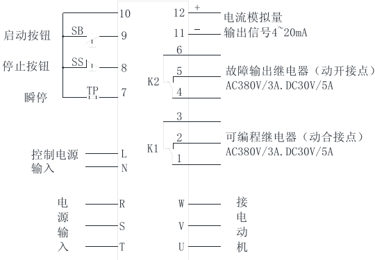
a. 起停分散控制接线图
