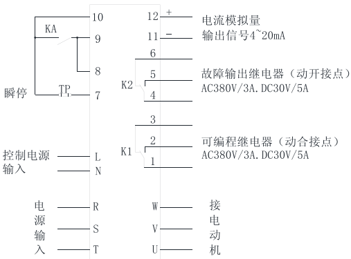
b. 起停合并继电器控制接线图
