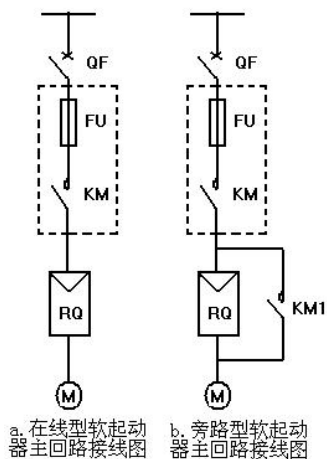
图4.1 主回路接线图
