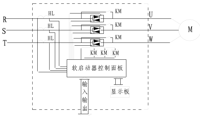
图 7.2 电气原理图 (75KW 以上)
