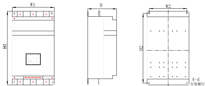
图 3.5 55KW 以上产品外形图
