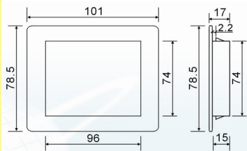
图 6.2 外接键盘开孔图
