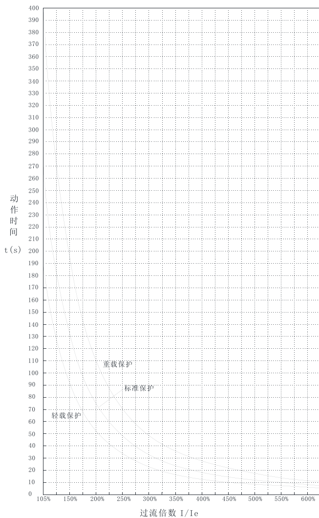
图5.2 软起动器热脱扣曲线（热态）
