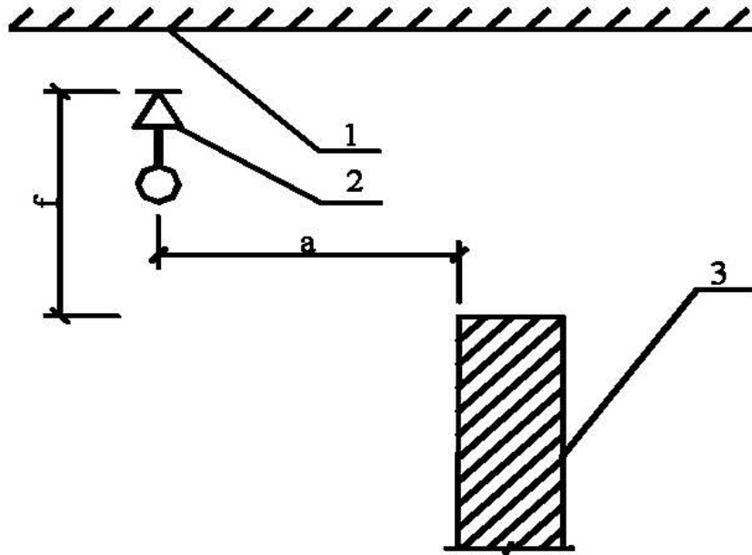
图 7.2.4 喷头与不到顶隔墙的水平距离
