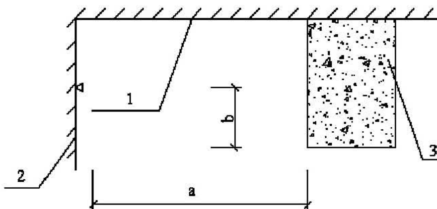
图 7.2.6 边墙型洒水喷头与正前方障碍物的距离
