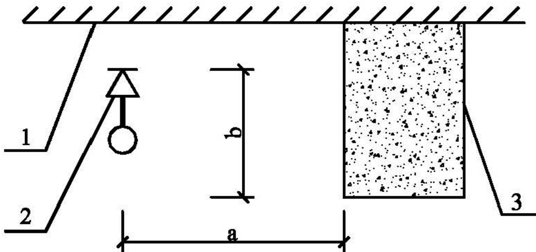
图 7.2.1 喷头与梁、通风管道等障碍物的距离
