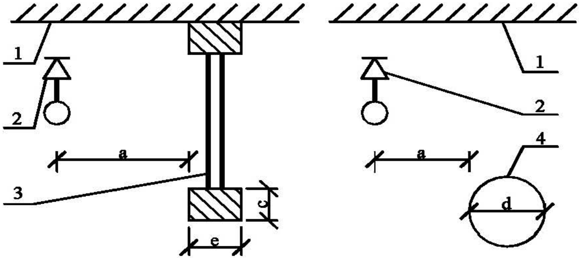
图 7.2.2 喷头与邻近障碍物的最小水平距离
