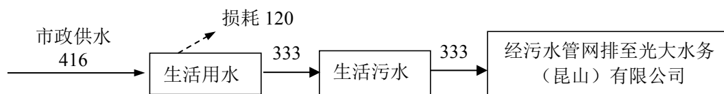
图 3.5-1 本项目全厂水量平衡图
