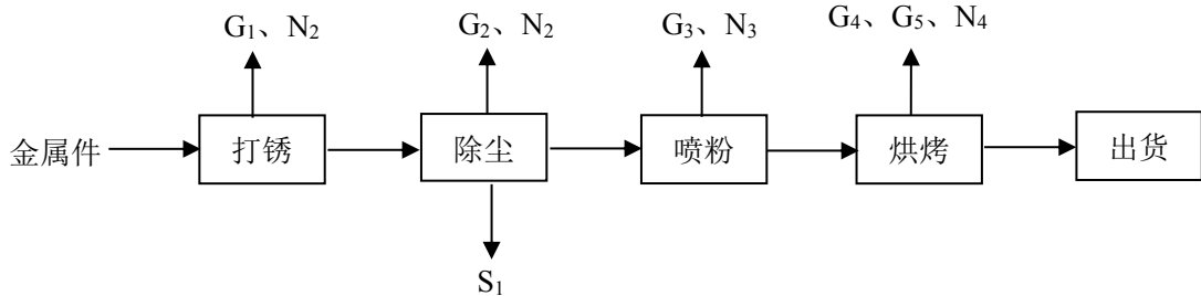
图 3.6-1 生产工艺流程
