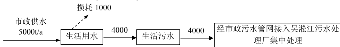
图 3.5-1 本项目厂区水量平衡图 ( \text{m}^3/\text{a} )
