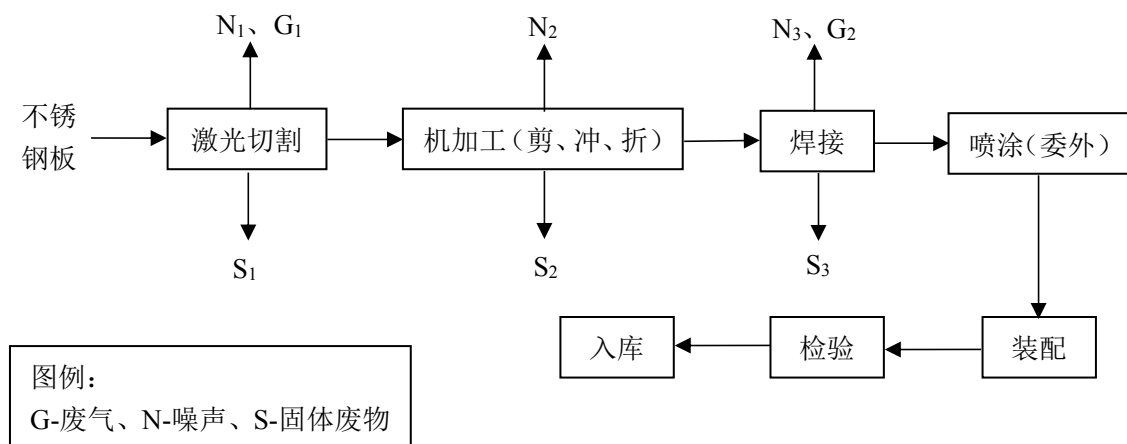
图 3.6-1 生产工艺流程图
