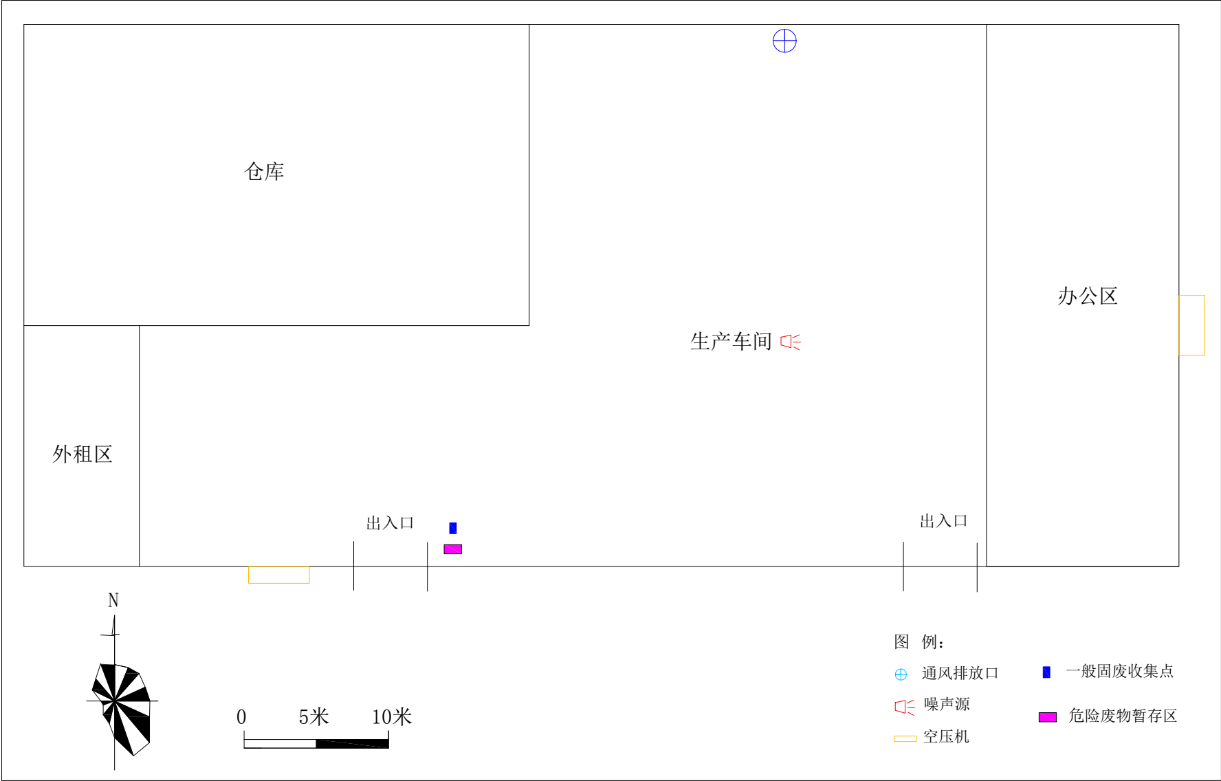
附图 4 项目厂房平面布置图
