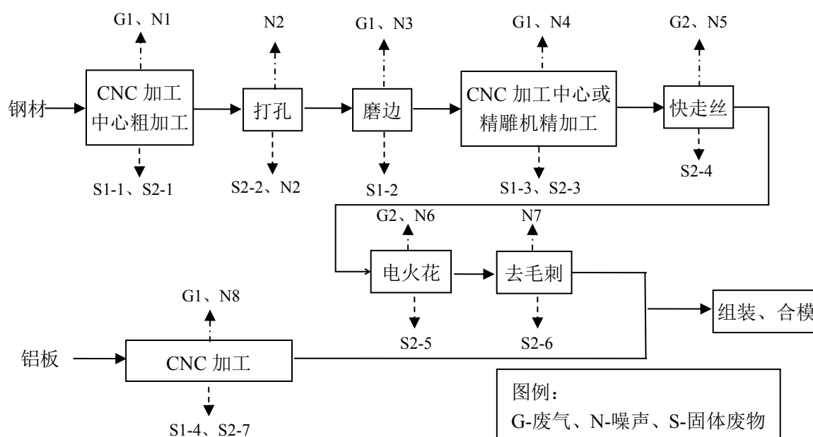
图 5-1 工艺流程图
