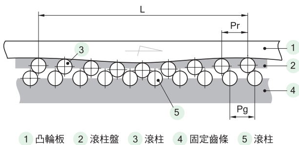
1 凸輪板 2 滾柱盤 3 滾柱 4 固定齒條 5 滾柱
