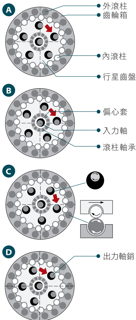
滾柱減速機的基本結構圖
