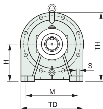
●單級臥式雙軸型 KHD 減速機尺寸表：
