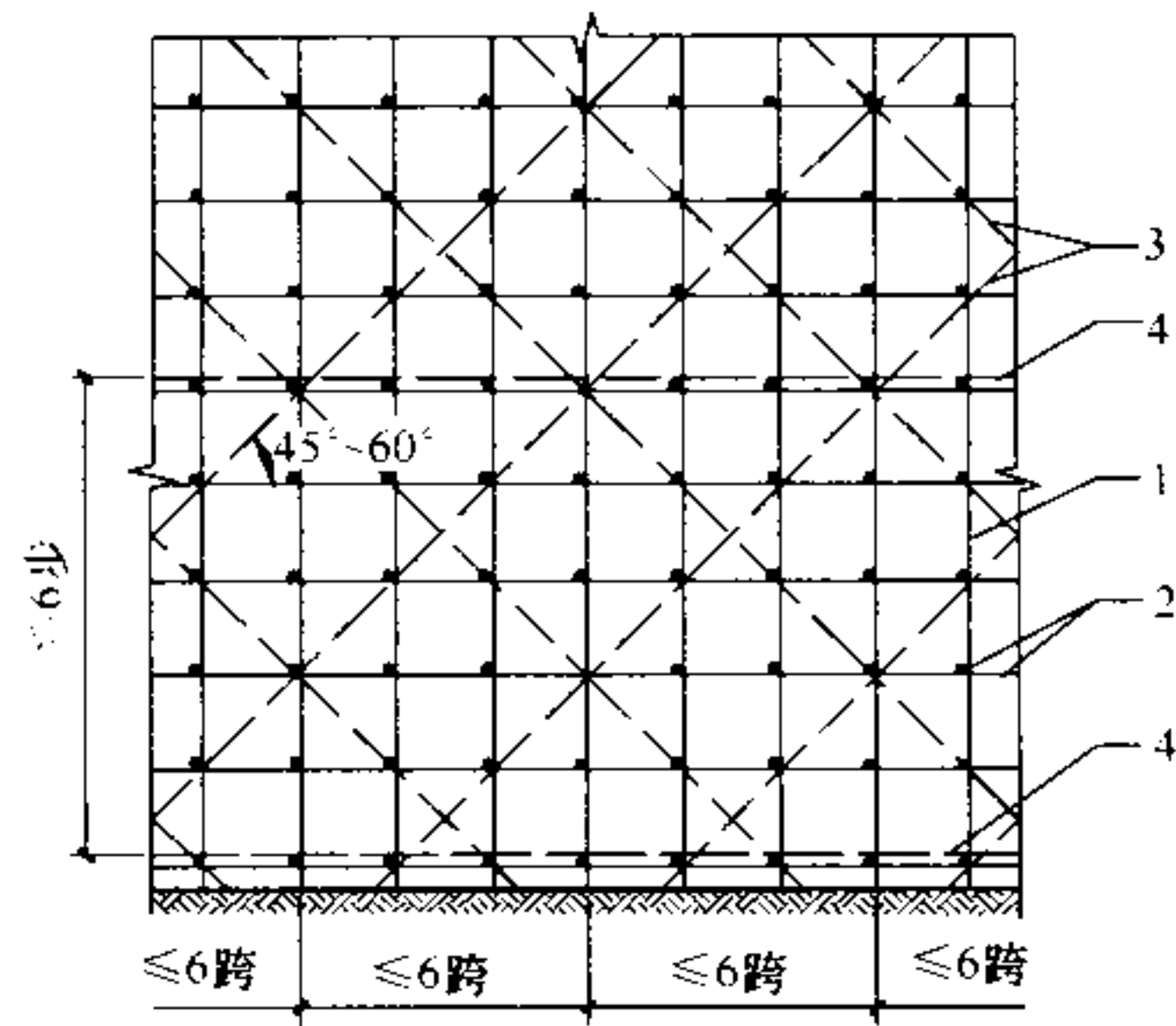
(b) 立面图
