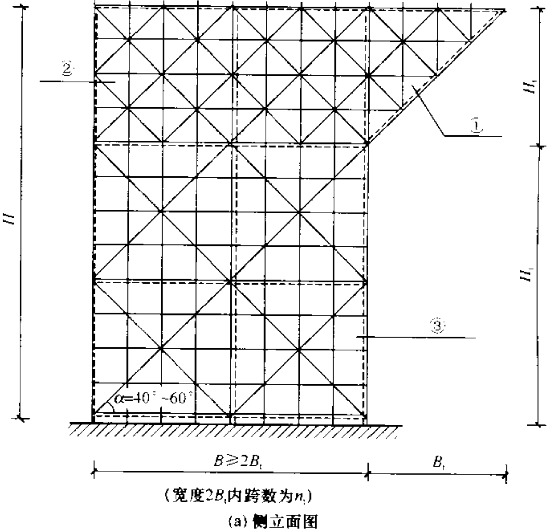
图 6.1.1 悬挑支撑结构示意图（一） ①—悬挑部分；②—平衡段；③—落地部分 注：虚线表示垂直于图面的剪刀撑或斜杆。
