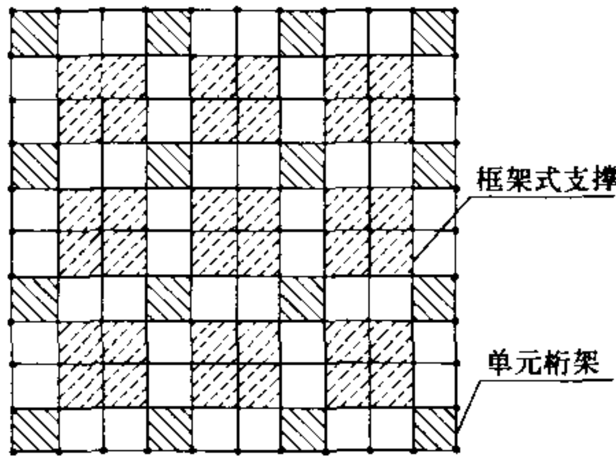
图 14 混合式支撑结构单元桁架布置方式
