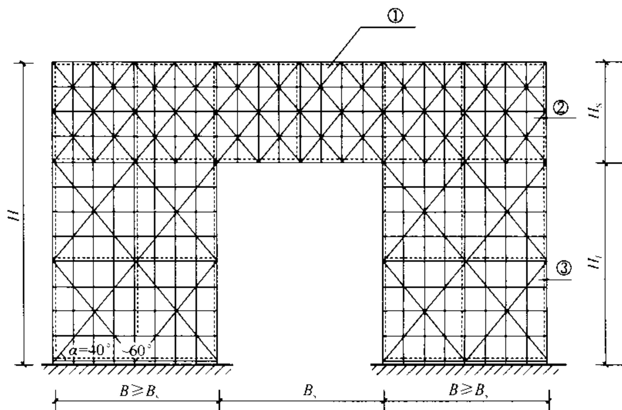
(a) 立面图
