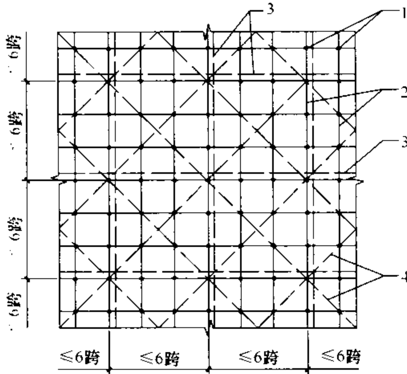
(a) 平面图
