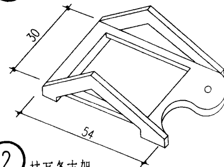
挂瓦条支架
