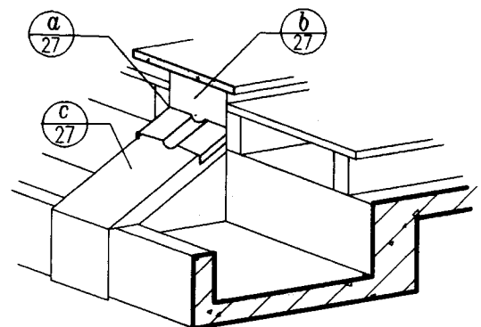
B 外天沟平直变形缝示意
