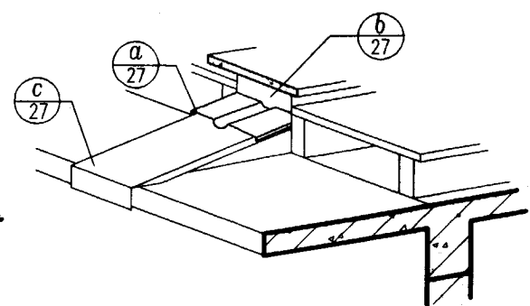
(未加盖板) A 挑檐平直变形缝示意
