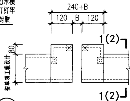
⑤ 女儿墙顶部平面 (未加盖板)
