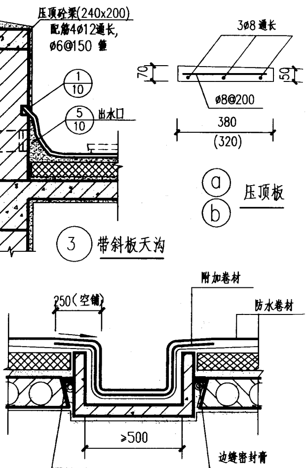
④ 预制屋面中天沟
