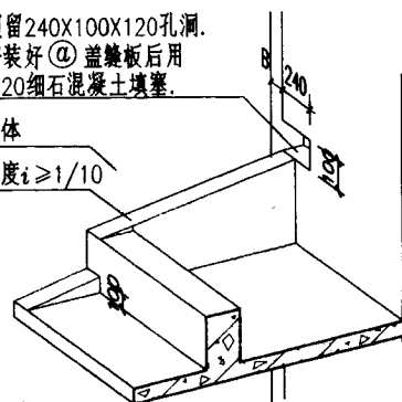
未加盖板示意图
