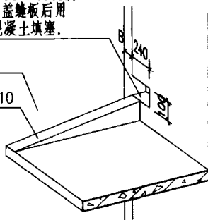
未加盖板示意图
