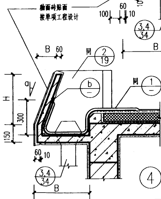
④ 带斜板天沟 (二)
