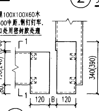
⑤ 女儿墙顶部平面 (未加盖板)
