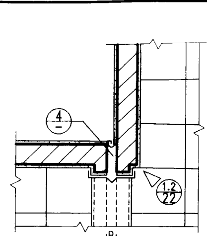
③ 女儿墙平面
