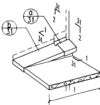
② 加金属盖缝板示意图
