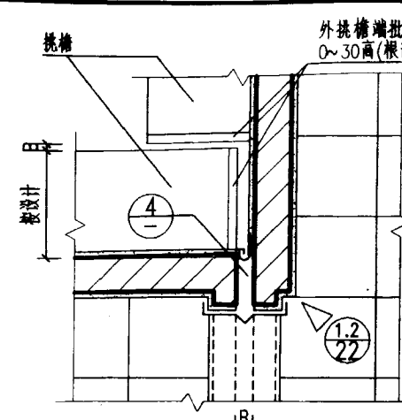
② 女儿墙(带外挑檐)平面
