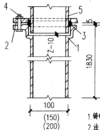
④ 柔性抗震接口
