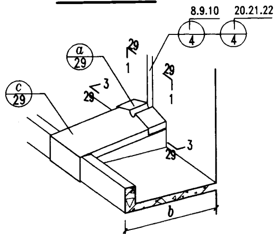
① 加金属盖缝板后示意图
