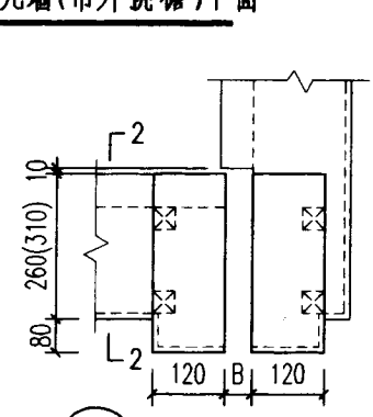
⑥ 女儿墙顶部平面 (未加盖板)
