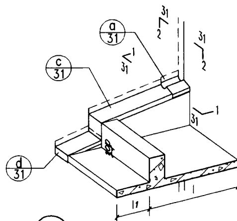
③ 加金属盖缝板示意图
