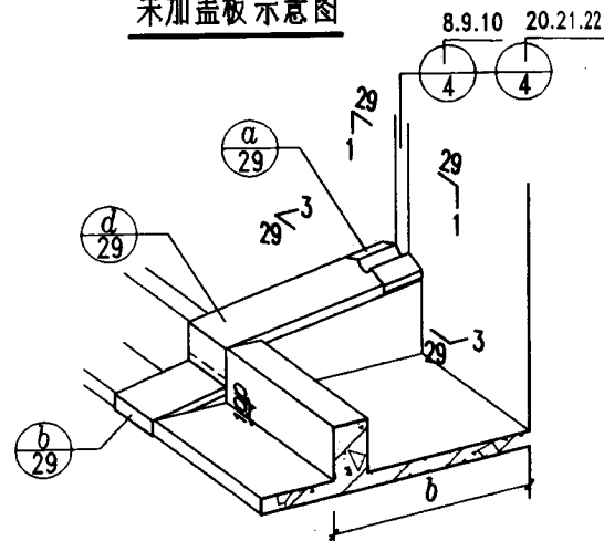
③ 加金属盖缝板后示意图
