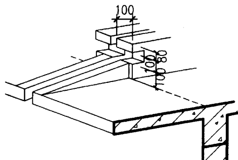
(未加盖板) A 挑檐平直变形缝示意
