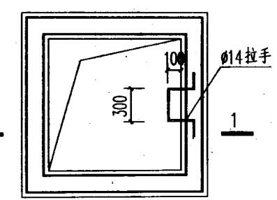
③ 钢筋砼检修孔
