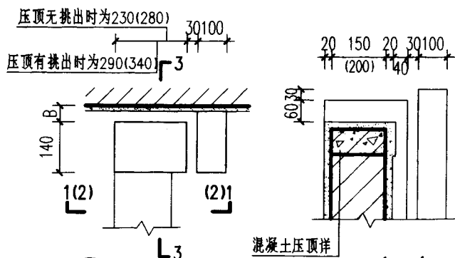
3 顶部平面
