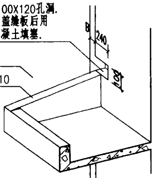
未加盖板示意图
