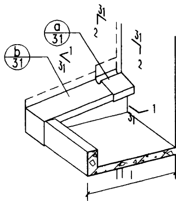
① 加金属盖缝板后示意图
