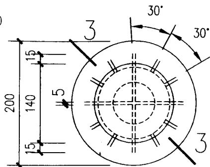
③ 铸铁罩
