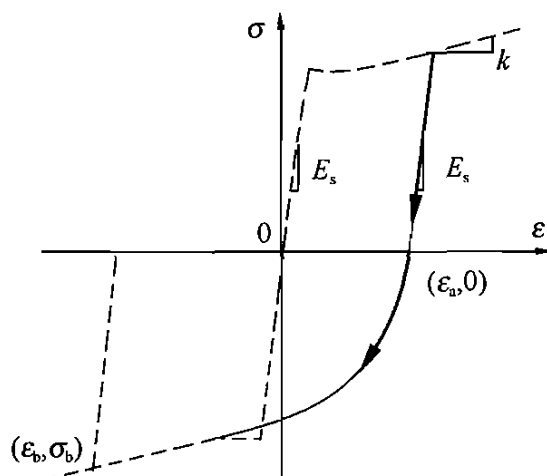
·图 C. 1. 3 钢筋反复加载应力-应变曲线
