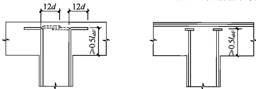
(e) 顶层中间节点柱筋90°弯折锚固
