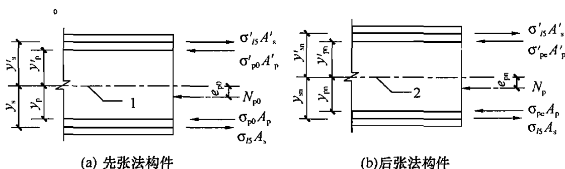
图 10.1.7 预加力作用点位置
