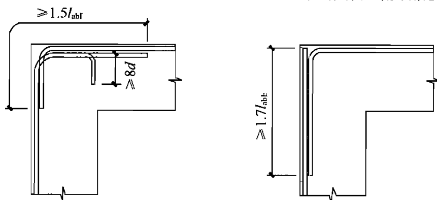
(g) 钢筋在顶层端节点外侧和梁端顶部弯折搭接
