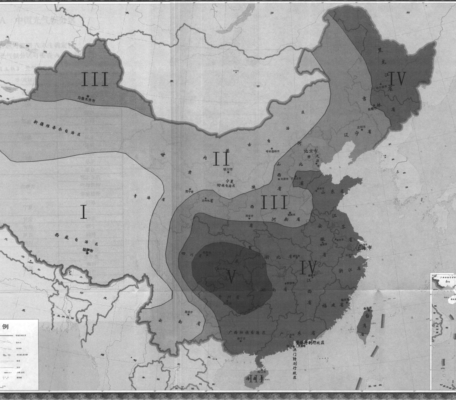
注：按天然光年平均总照度 (klx)：I. E_q \geq 45 ；II. 40 \leq E_q < 45 ；III. 35 \leq E_q < 40 ；IV. 30 \leq E_q < 35 ；V. E_q < 30 。
